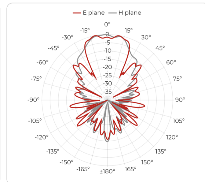
6 GHz
