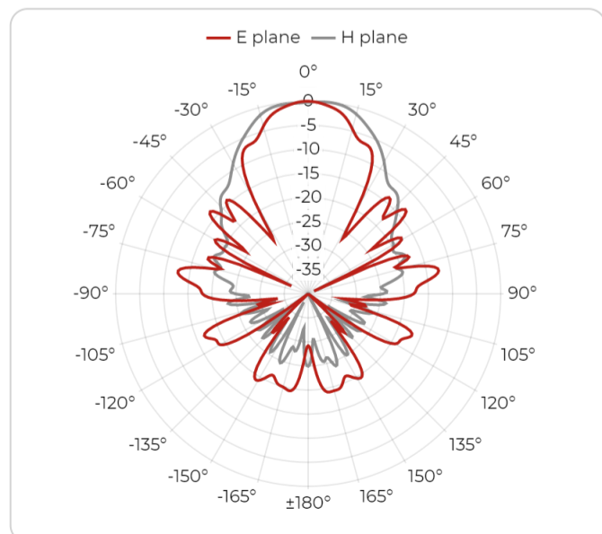
5 GHz
