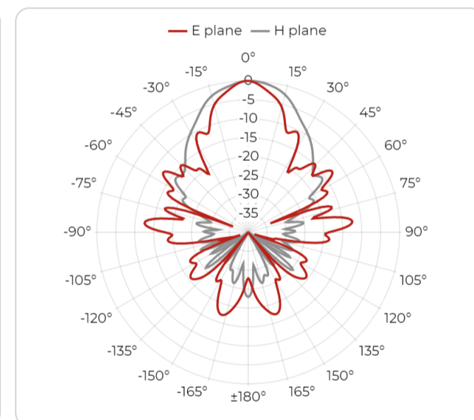
4.5 GHz
